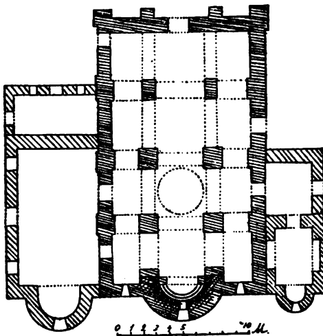
Приблизительный планъ церкви Παναγία Ἀγυιόκτιστος.
